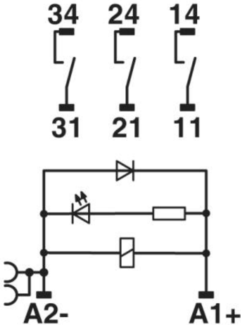
Diagrama eléctrico
