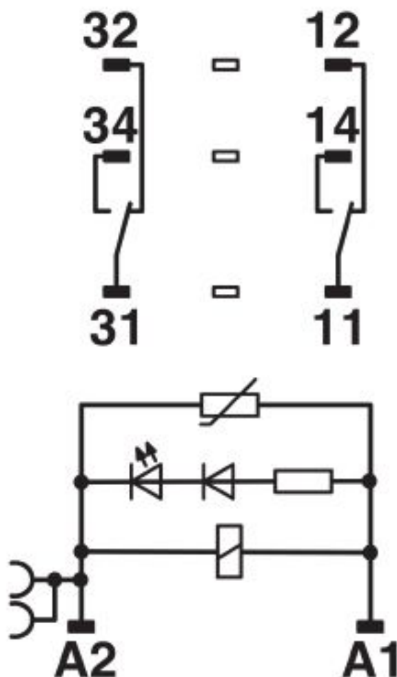
Diagrama eléctrico
